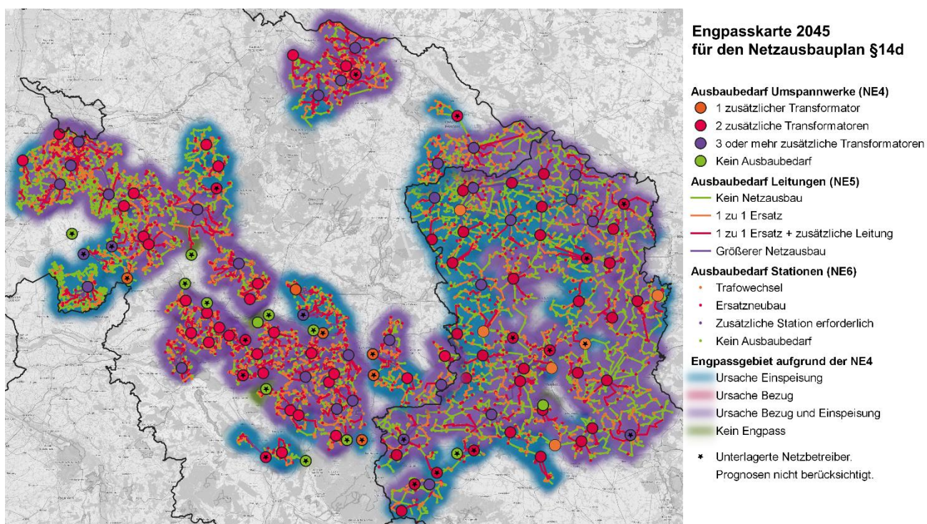
Abbildung 6: Engpasskarte 2045 gesamtes Mittelspannungsnetzgebiet Avacon
