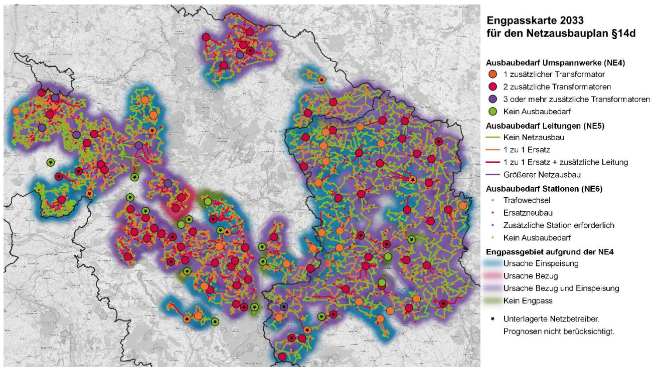
Abbildung 5: Engpasskarte 2033 gesamtes Mittelspannungsnetzgebiet Avacon
