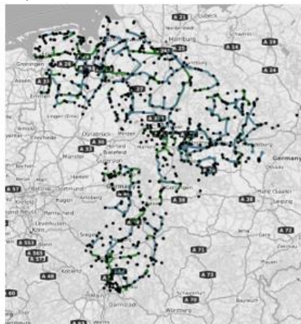
Abbildung 3: Darstellung der Engpässe im HS-Netz der Avacon nach Jahresscheibe
